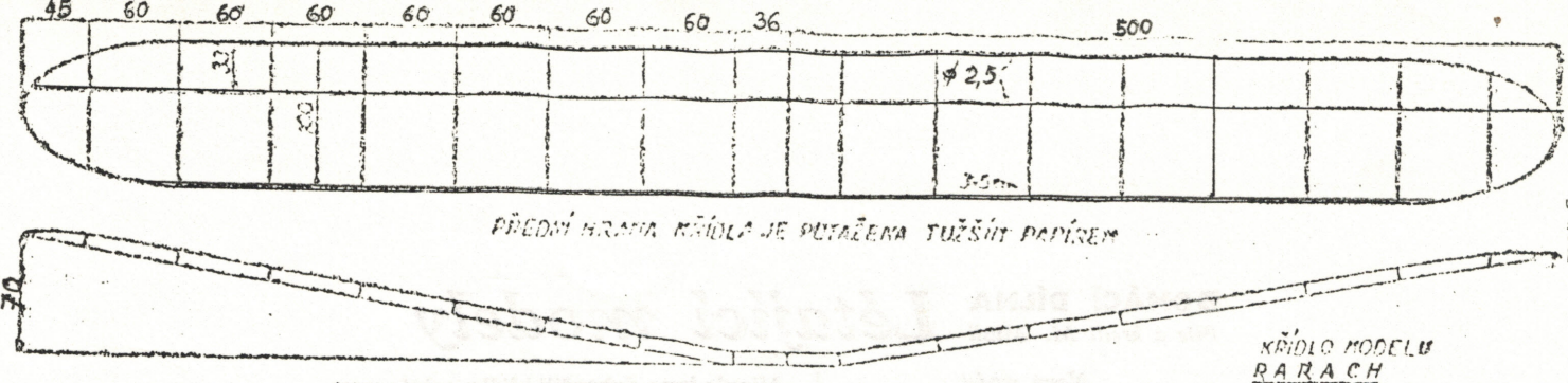
Křídlo modelu „Rarach“ zmenšeno na 1:110.
